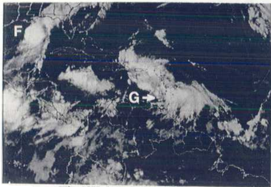
p) 1303 9 September 1988
