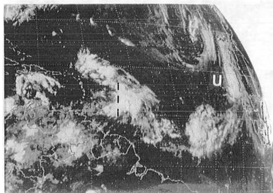
l) 1201 8 September 1988
