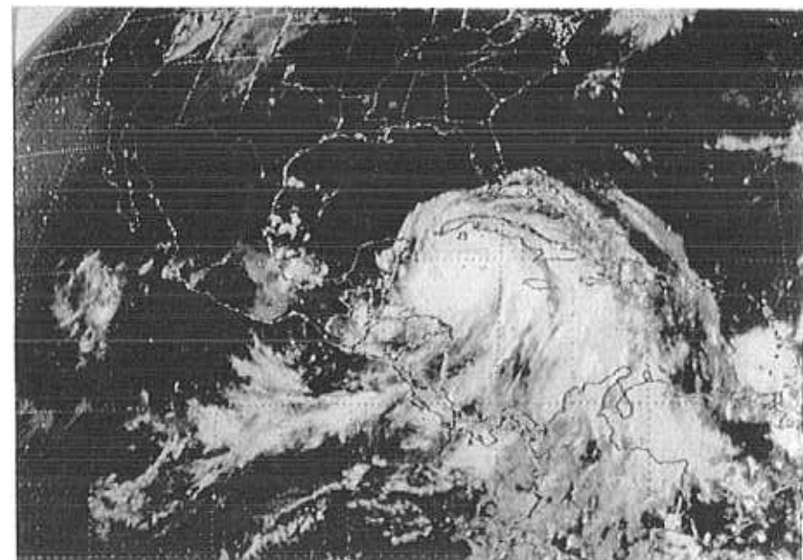
gg) 1801 13 September 1988
