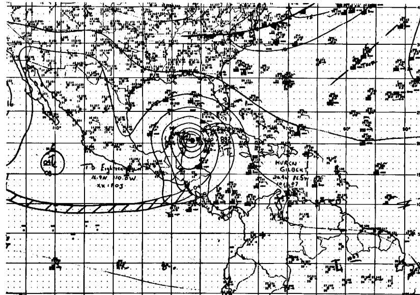
x) 1200 14 September 1988
