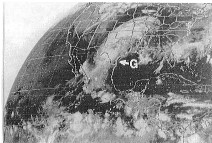
yy) 0701 18 September 1988
