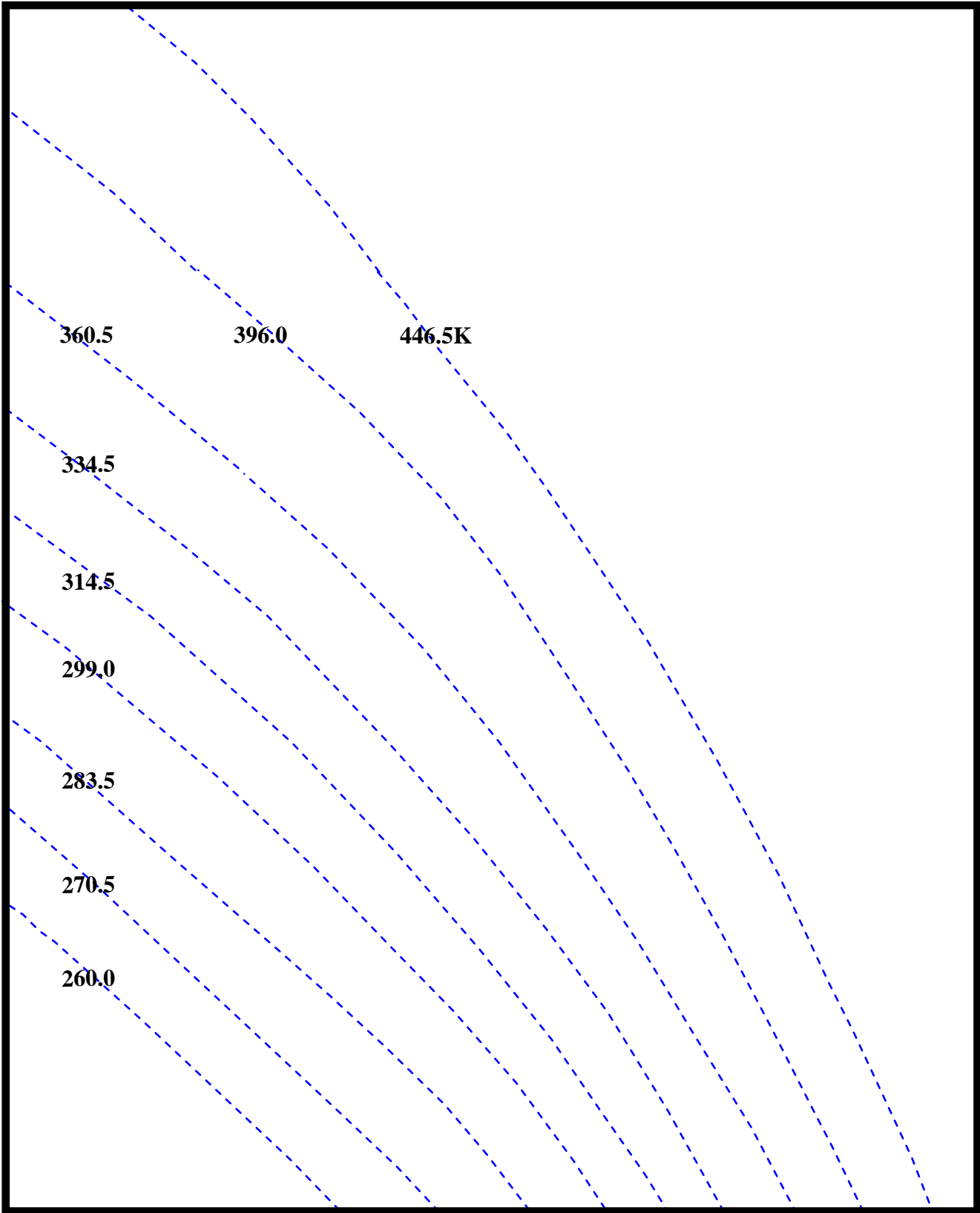
Wet Adiabats (Kelvin)
