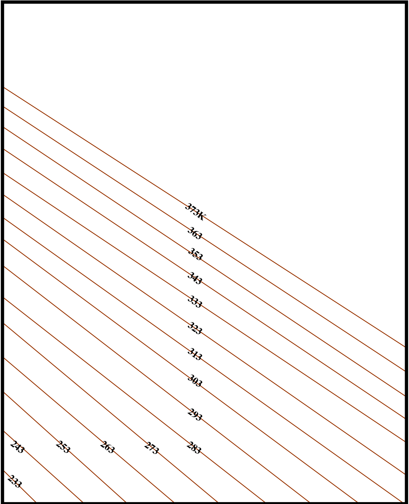
Dry Adiabats (Kelvin)
